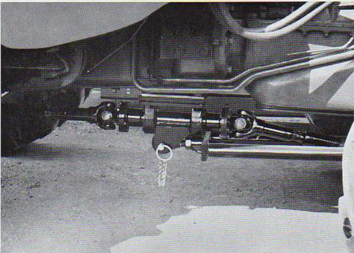
Zwischenlager mit Kardanwellen
