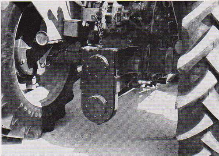
Aufsteck-Kettengetriebe an der hinteren Zapfwelle
